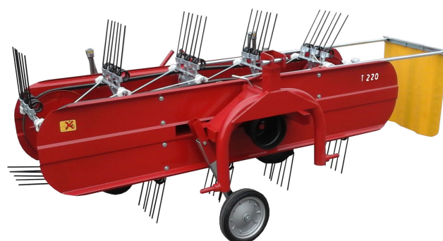
Abb. 2 Bandschwader T 200
