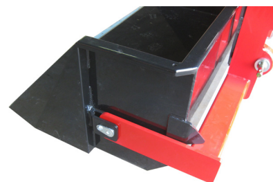
Fig. 3 Dettaglio sistema di sgancio MEC MINI/MIDI con perno di sicurezza Unhooking system detail MEC MINI/ MEC MIDI with safety pin
