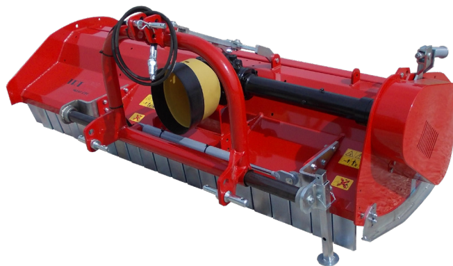
Fig. 2 Dettaglio rotore con mazze per TRT MAXI (Peso mazza Kg.1,35) Hammers rotor detail for TRT MAXI (Hammer weight 1,35 Kg)
