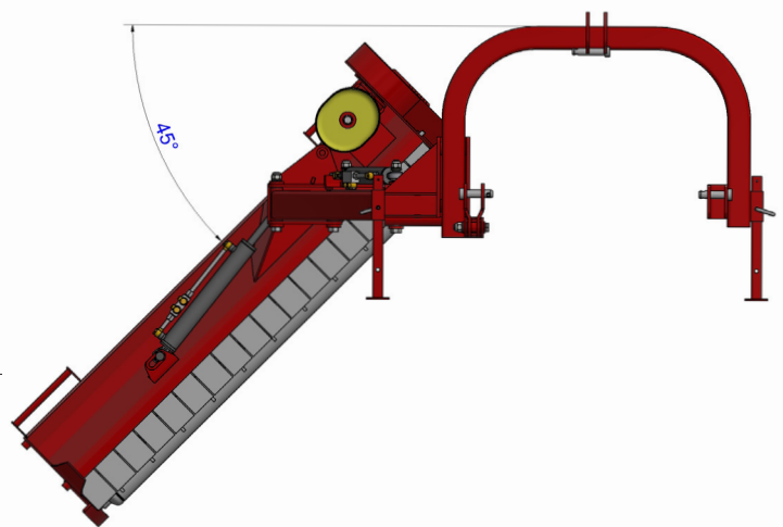
Abb. 2 Schlegelmäher TRL-M in ausgefahrener und geneigter Position
