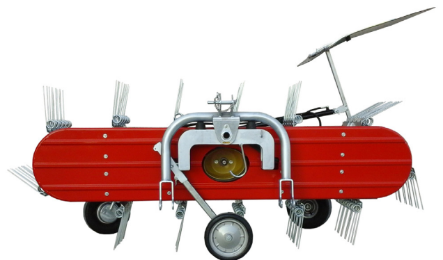
Abb. 7 Dreieck-Anschluss mit Stange und Tastrad
